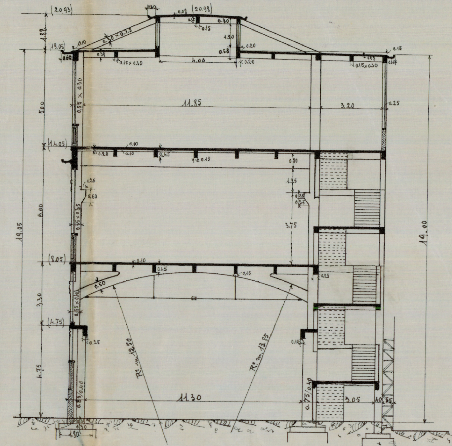
= SEZIONE TRASVERSALE "A-B" = Scala \frac{1}{100} =
